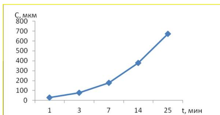
Рис. 5. График изменения конусности от времени обработки
