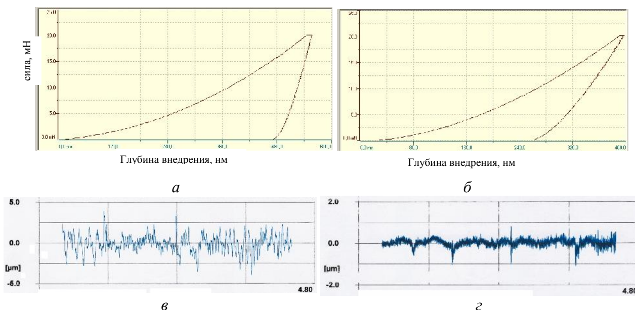
Рис. 2 Кривые наноиндентирования (а, б) и профилограммы (в, г) на поверхности титана: а – до УЗО; б – после УЗО.
