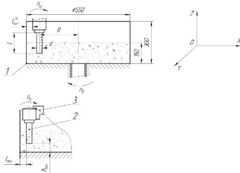
Рис. 2. Принципиальная схема обработки
