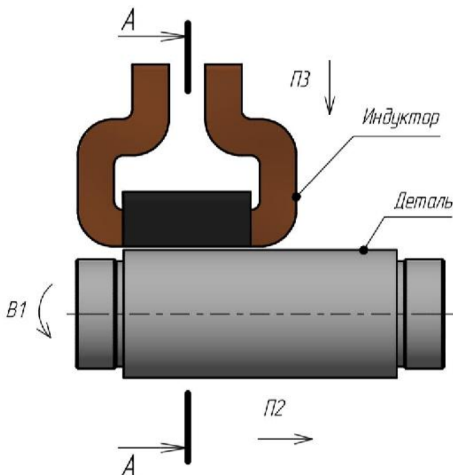
Рис. 1. Процесс ВЭН ТВЧ
