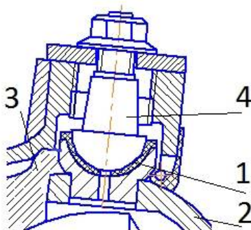
Рис. 1. Заводская конструкция поворотного кулака автомобиля УАЗ: 1 – опора полусферическая; 2 – корпус поворотного кулака; 3 – ШОПК; 4 – шкворень
