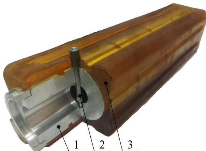
Рис. 1. Конструкция сборочной единицы
