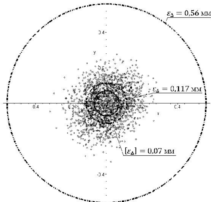
Рис. 4. Диаграмма отклонений суммарного эксцентриситета
