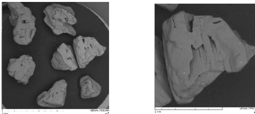
Рис. 1. Зёрна абразивного материала – электрокорунд
