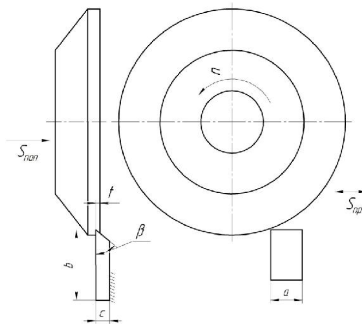
Рис.1. Принципиальная схема затачивания пластины
