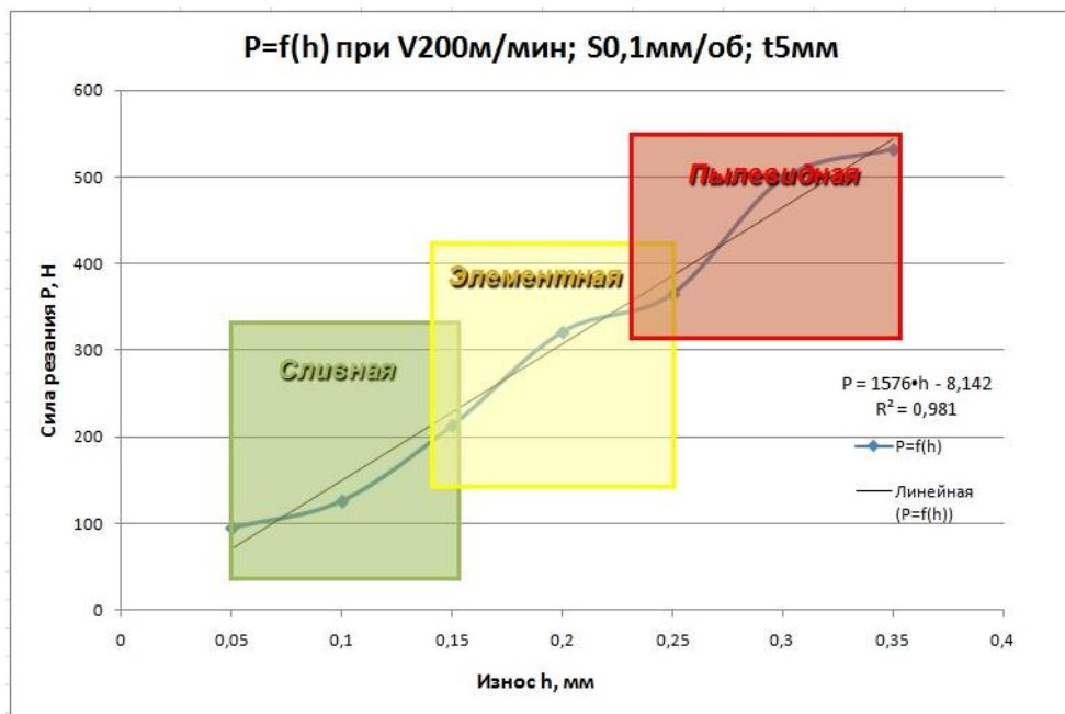
Рис. 2. График зависимости изменения типа стружки от износа режущего инструмента и силы резания
