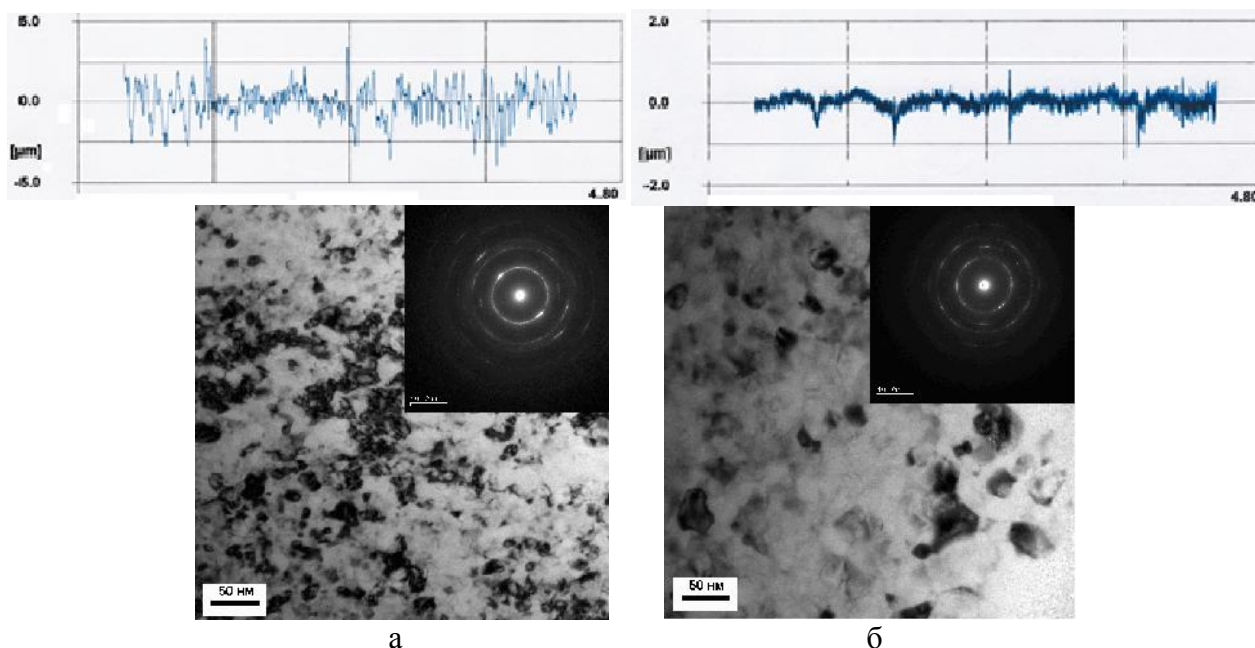
Рис. 3. Микроструктура наноструктурного никелида титана после УЗО ( P_{ст}=100 Н) на поверхности (а) и на глубине ~14 мкм от поверхности (б).
