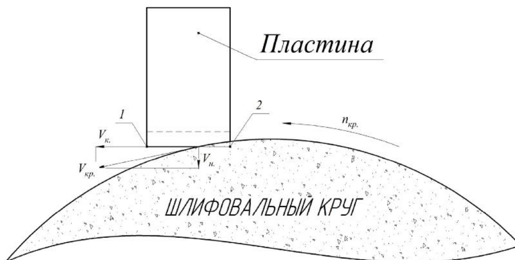
Рис.2. Принципиальная схема задания скорости сдвига.
