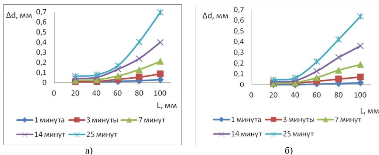
Рис. 4. Изменения диаметра образцов:
