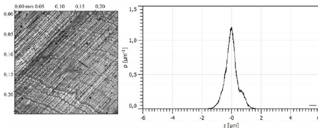
Рис. 2. Деформационный рельеф (а), график функции плотности распределения ординат (б), \text{Ni} , e=20\% , следы сдвига
