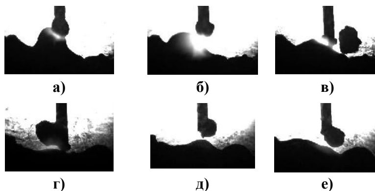
Рис. 3. Видеокадры плавления и переноса электродного металла в сварочную ванну различных интервалов сварочного микроцикла с применением CuBr -лазера.
