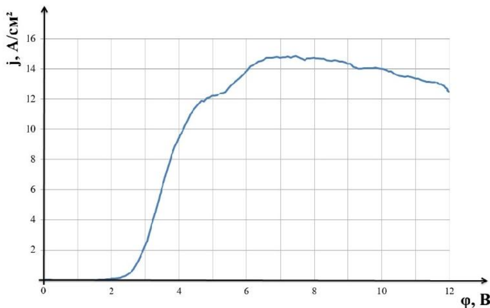
Рис.2. Потенциодинамическая поляризационная кривая анодного растворения сплава 5БДСР в 10% водном растворе сульфата натрия
