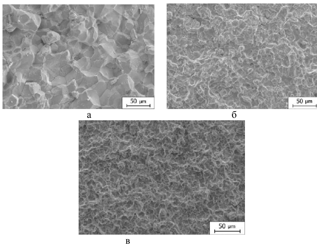
Рис. 5. Изломы эвтектоидной стали с мартенситной структурой: после ХТО (1000 °С, 6 ч.) (а); после ХТО и отжига по режиму: выдержка при 740–760 °С, охлаждение с печью до 600 °С (б); после ХТО, 3 циклов ТЦО (в)
