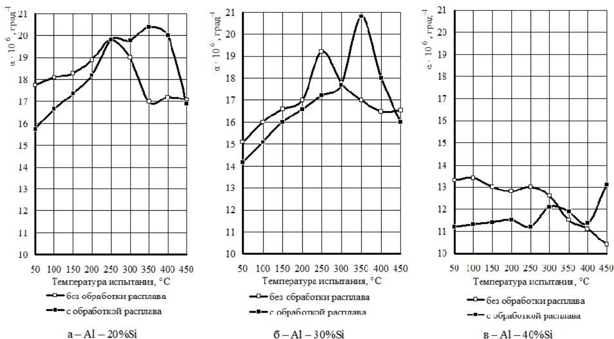
Рис. 1. Влияние обработки расплава парами водного раствора \text{CuSO}_4 на линейное расширение сплавов Al-Si
