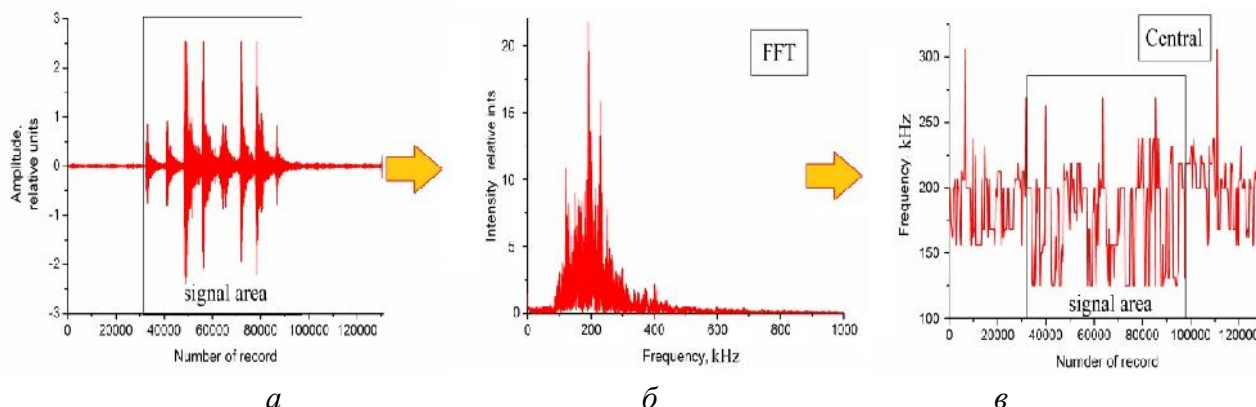
Рис. 1. Характерный сигнал АЭ в области установившегося трения [10 \overline{7} 1] – монокристаллов
