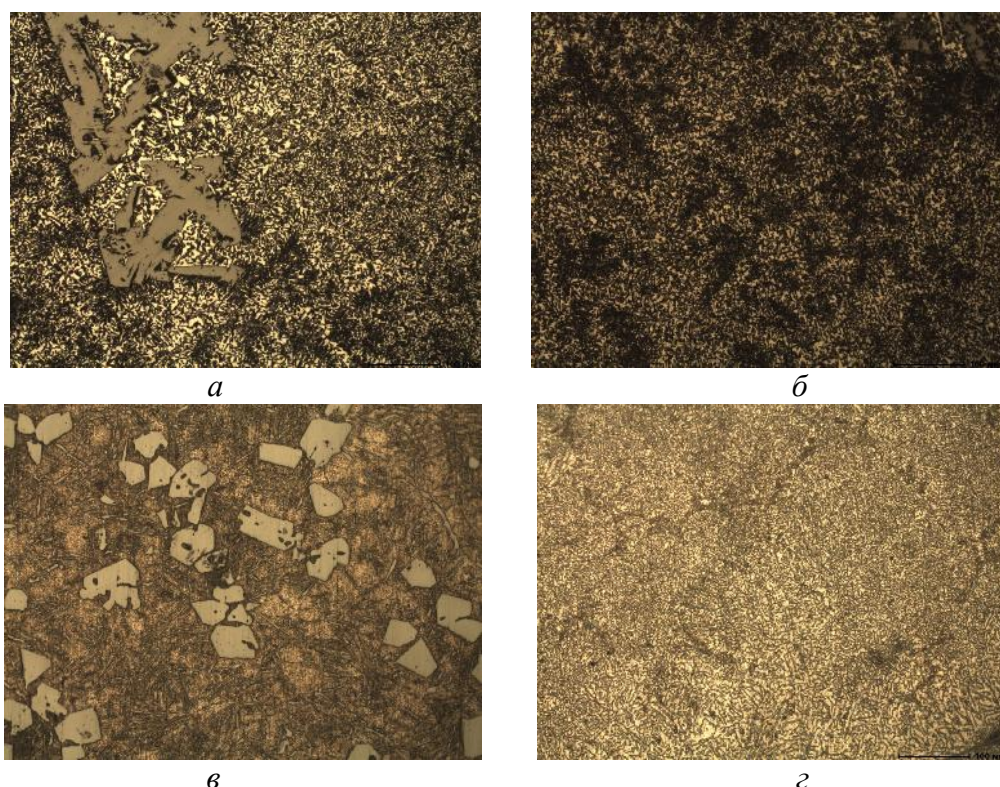
Рис. 2. Микроструктура сплава Al – 20% Si:
