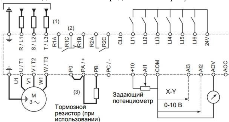
Рис. 2. Схема подключения электропривода
