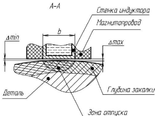
Рис. 2. Сечение А-А рисунка 1
