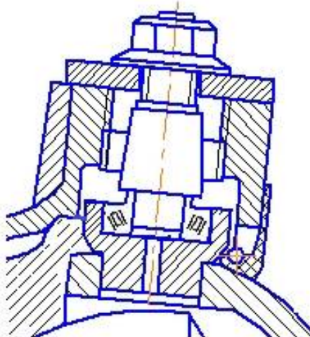
Рис.2. Модернизированный шкворневый узел с подшипником качения
