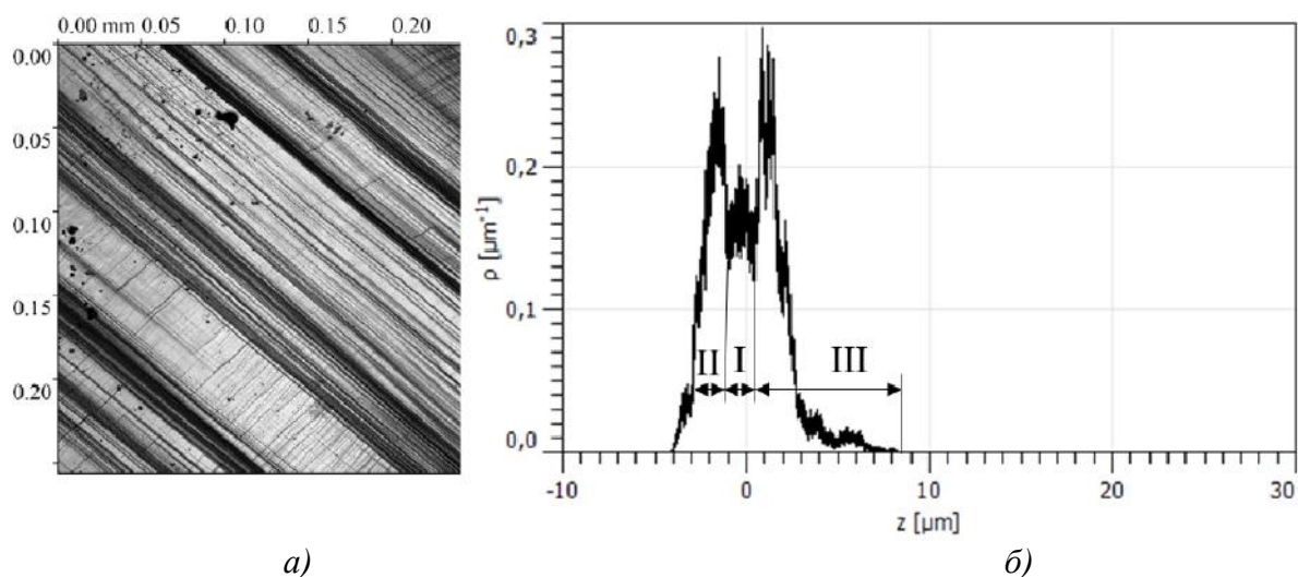
Рис. 1. Деформационный рельеф (а), график функции плотности распределения ординат \text{Ni}_3\text{Fe} БП (б), e=20\% , пачки следов
