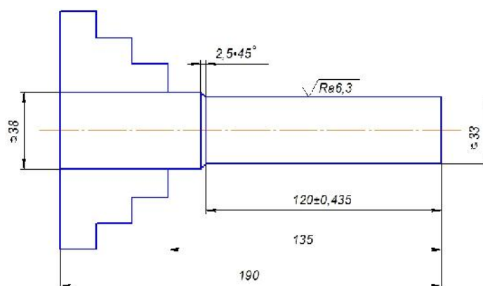
Рис. 1. Эскиз детали
