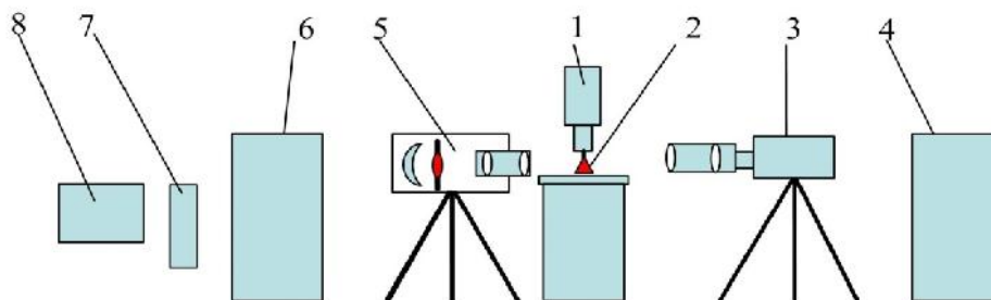
Рис. 1. Исследовательский комплекс:
