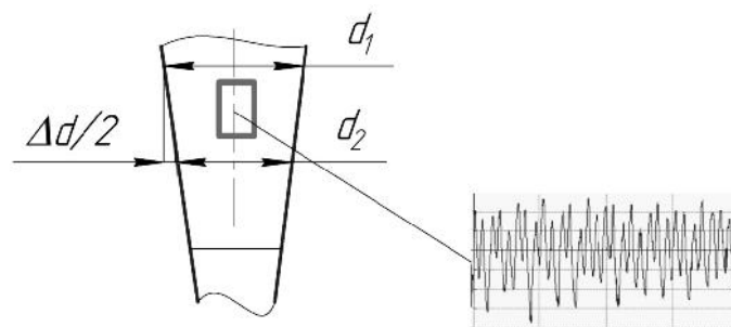
Рис. 3. Схема контроля изменения диаметра и шероховатости поверхности
