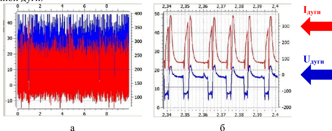
Рис. 4. Осциллограммы тока и напряжения дуги при работе лазера в режиме видеосъемки: а – до обработки, б – после обработки изображений
