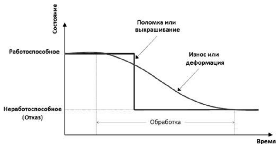
Рис. 1. Виды неисправностей режущего инструмента
