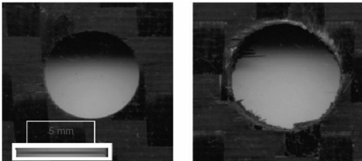
Рис. 1. Профиль отверстия в углепластике при различной величине подачи. [2]
