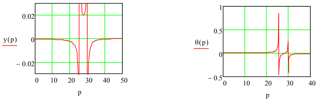
Рис. 2. Зависимости y(p) и \theta(p) от частоты
