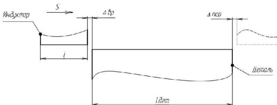
Рис. 3. Поверхностная закалка ВЭН ТВЧ «на проход»
