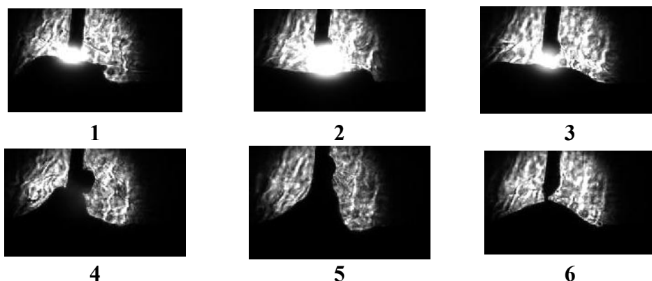
Рис. 2. Видеокадры сварочного микроцикла (период плавления и переноса одной капли электродного металла), последовательность кадров: 1 - 2 - 3(интервал горения дуги), 4 -5 -6 (интервал короткого замыкания).
