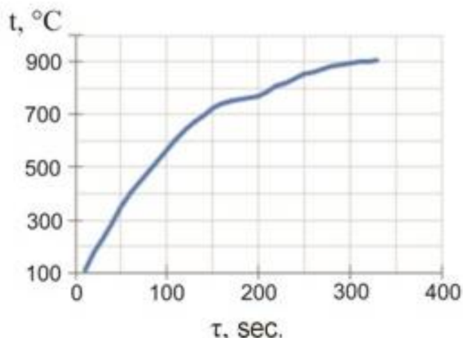
Рис. 2. График нагрева образца из эвтектоидной стали в печи, нагретой до 900 °C
