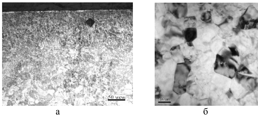
Рис 1. Вид микроструктуры Ti в поперечном сечении после УЗО: а – оптика; б – ПЭМ
