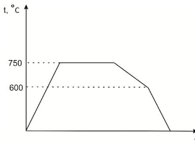
Рис. 1. График изотермического отжига эвтектоидной стали на зернистый перлит
