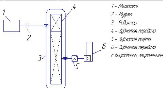
Рис.1. Кинематическая схема
