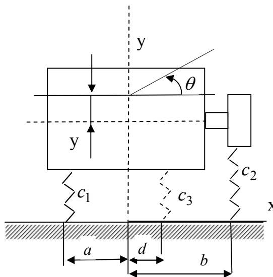
Рис.1. Схема подвески дизель-генератора (2-е степени свободы)
