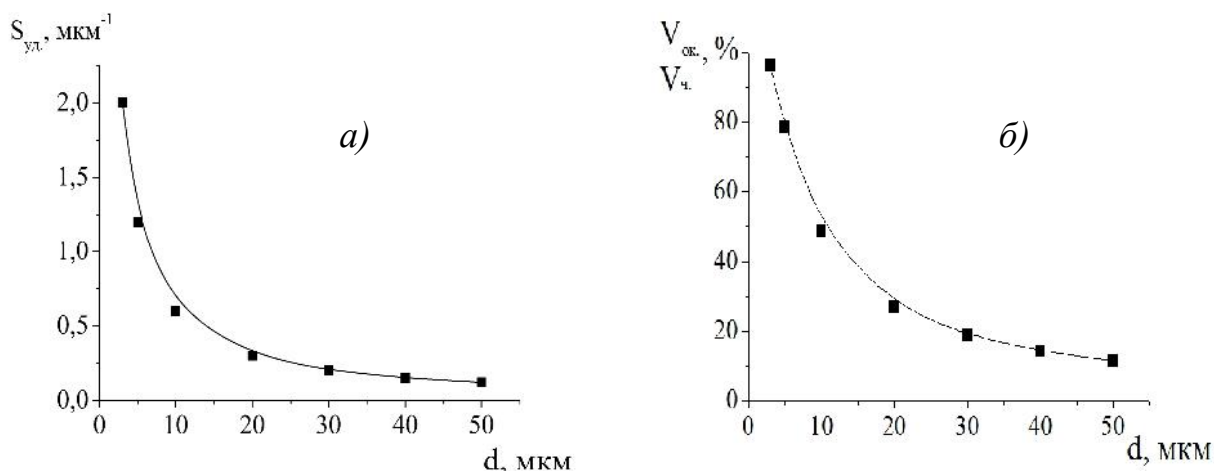
Рис. 7. Зависимость удельной площади поверхности ( S_{уд}=S_{ч}/V_{ч} , где S_{ч} – площадь поверхности частицы; V_{ч} – объем частицы) (а) и удельного окисленного объема V_{ок}/V_{ч} (б) от размера d напыляемых частиц
