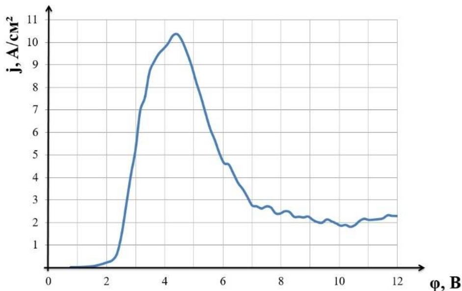
Рис.1. Потенциодинамическая поляризационная кривая анодного растворения сплава 5БДСР в 10% водном растворе нитрата натрия
