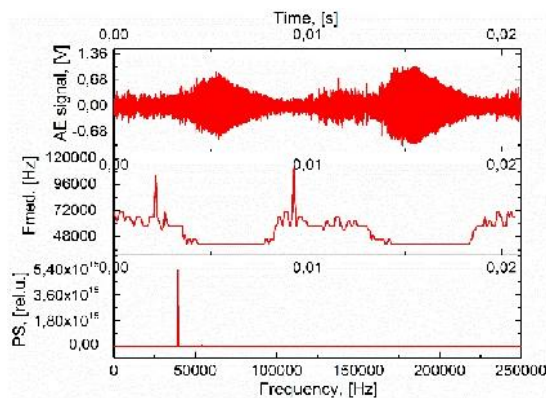
Рис. 2. Фрейм сигнала АЭ, его медианная частота и мощность спектра после 48 часов трения
