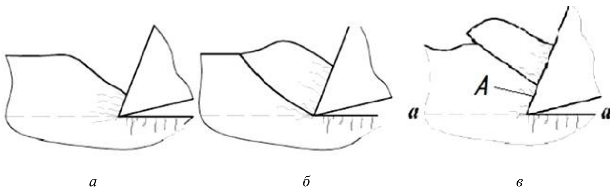
Рис. 1. Процесс образования стружки при резании композиционного материала: а, б, в – последовательные стадии стружкообразования [1, 10]
