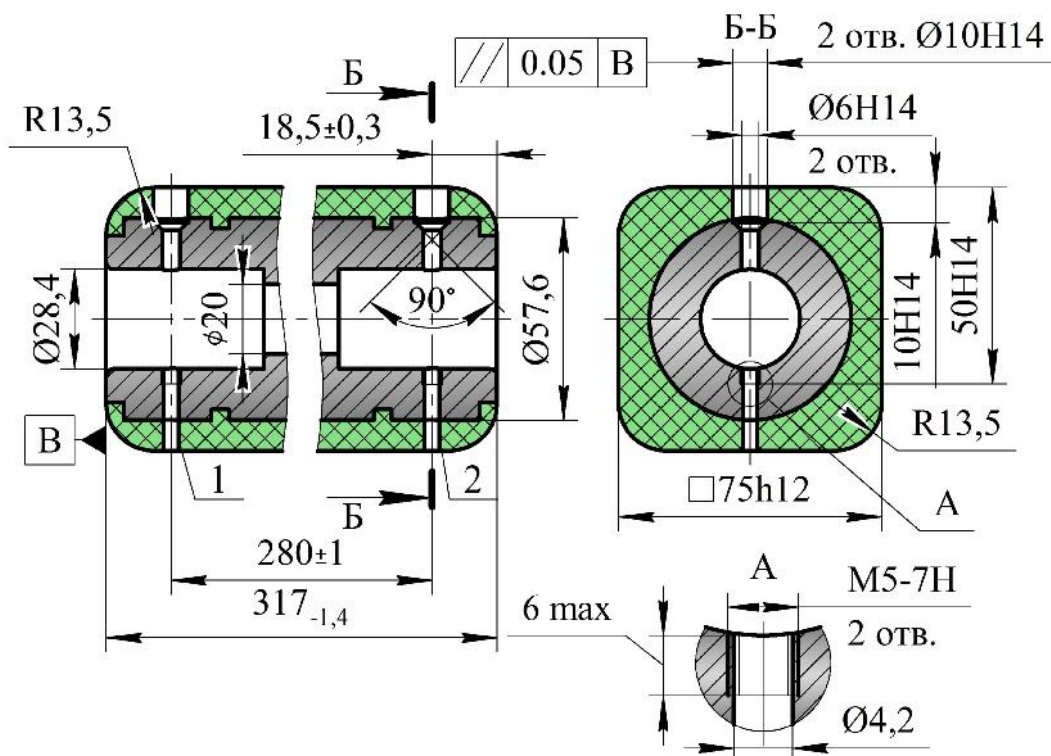
Рис. 2. Наличие глубоких отверстий в сборочной единице
