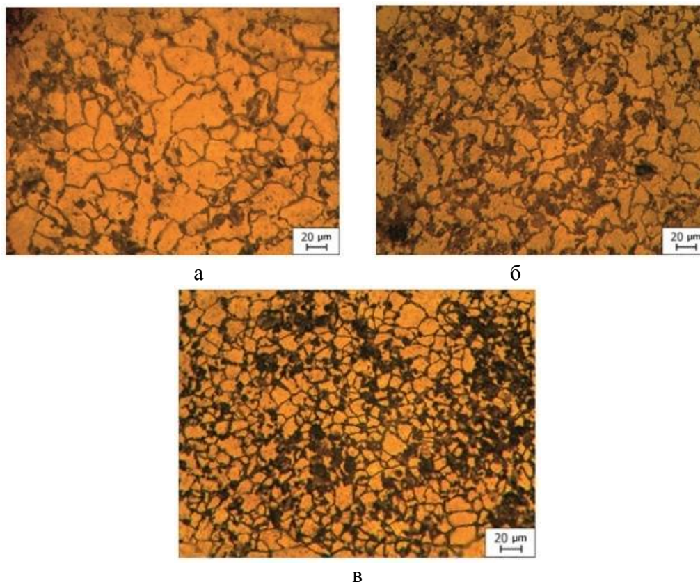
Рис. 4. Микроструктура эвтектоидной стали с трооститной сеткой (ГОСТ 5639-82): после ХТО (1000 °С, 6 ч.) (а); после ХТО и отжига по режиму: выдержка при 740–760 °С, охлаждение с печью до 600 °С (б); после ХТО, 3 циклов ТЦО (в).
