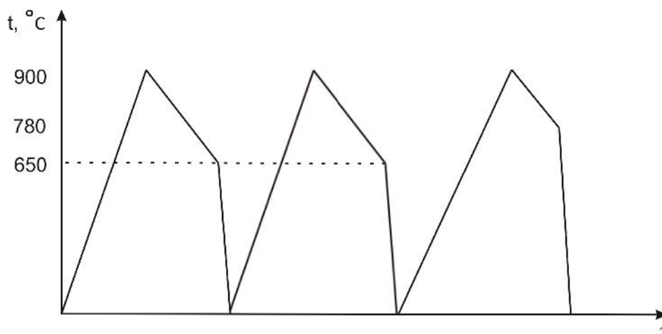
Рис. 3. График термоциклирования с закалкой эвтектоидной стали
