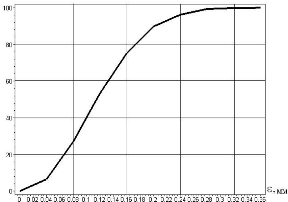
Рис. 5. Интегральная кривая процентного распределения значений суммарного эксцентриситета
