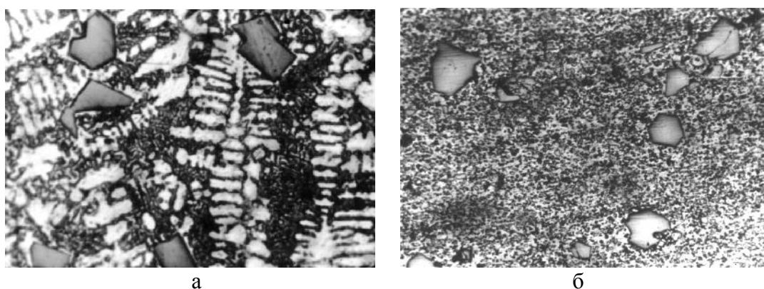
Рис. 1. Микроструктура слитка (а) и прессованного прутка (б) из легированного заэвтектического силумина
