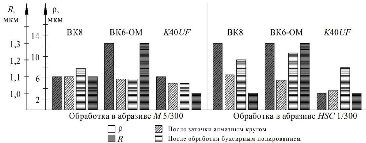
Рис. 3. Изменение радиуса округления \rho и шероховатости R режущих кромок твёрдосплавных пластин
