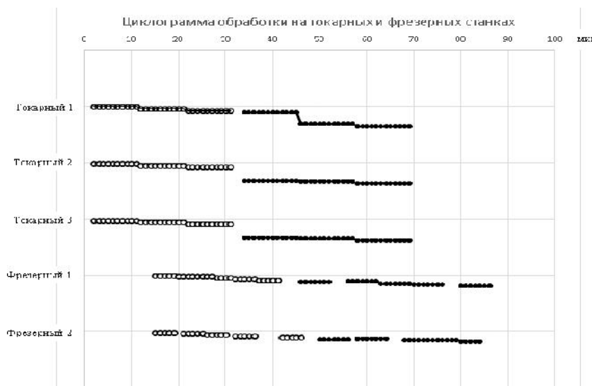
Рис. 3. Циклограмма обработки партий двух деталей на токарных и фрезерных станках при последовательном запуске (белым – график обработки первой детали; черным – график обработки второй детали)
