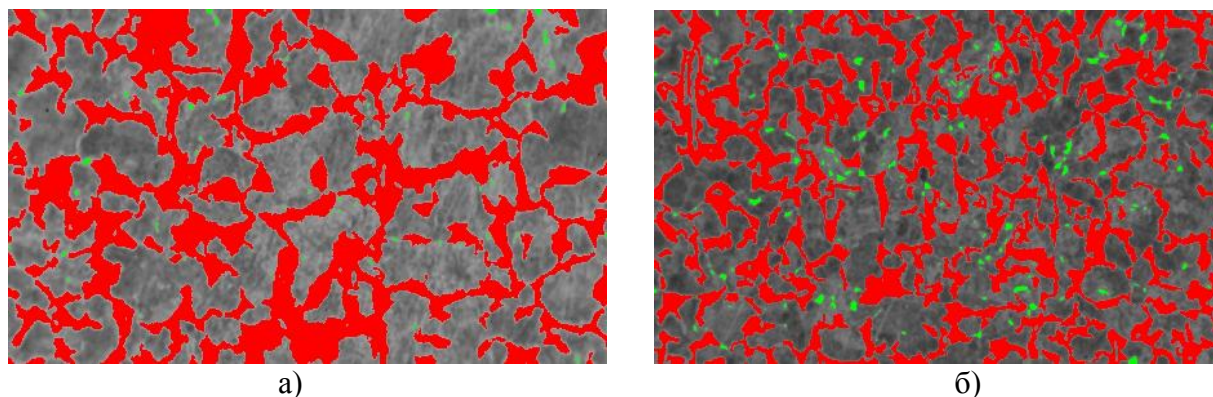
Рис.2. Количественный анализ структурных элементов при охлаждении в сыпучем графите (а) и на воздухе (б), ( \times 400 )
