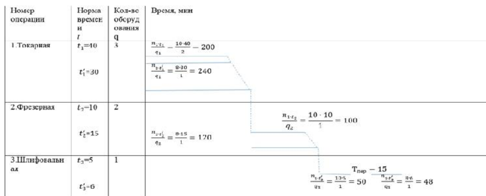
Рис. 2. Параллельно-последовательный запуск партий деталей в производство [3]
