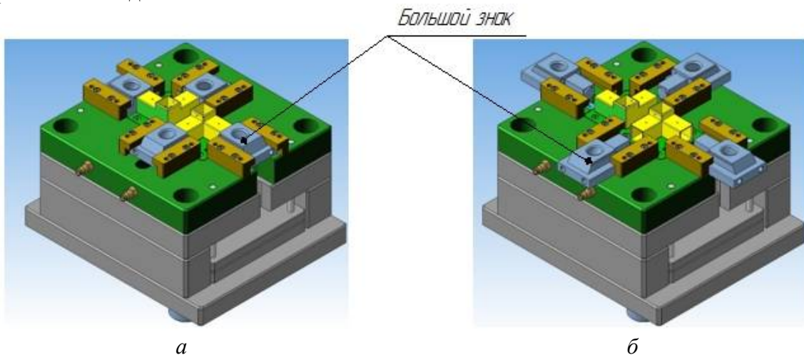
Рис. 2. Пресс-форма: а - положение 1; б - положение 2
