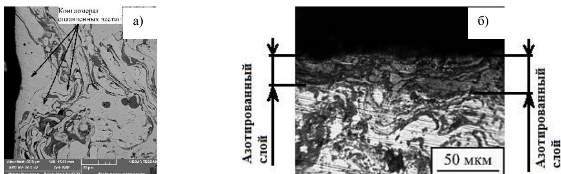
Рис. 2. Характерные микроструктуры газотермического покрытия из стали 40X13: а – исходное состояние; б – после ионно-лучевого азотирования при 870 К (3 часа)
