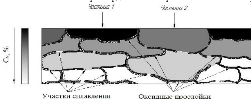
Рис.4. Схема имплантированного ионами азота участка поверхностного слоя газотермического покрытия с частицами различного размера (частицы более темного цвета имеют повышенную концентрацию атомов азота) [5]
