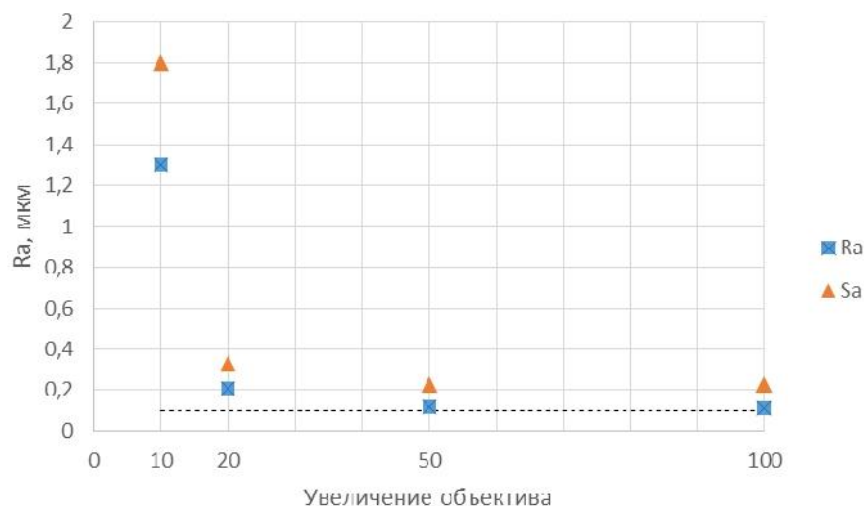
Рис. 1. Зависимость значений параметров шероховатости от увеличения объектива, пунктирной линией указано значение для образца шероховатости Ra=0,1 мкм
