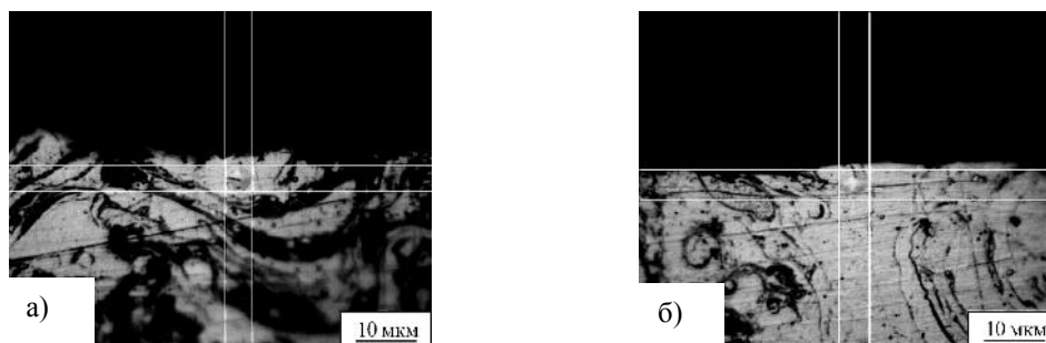
Рис. 5. Микроструктуры обработанного ионами азота ( T=870 К, 3 часа) газотермического покрытия из стали 40X13 с нанесенными отпечатками Виккерса:
