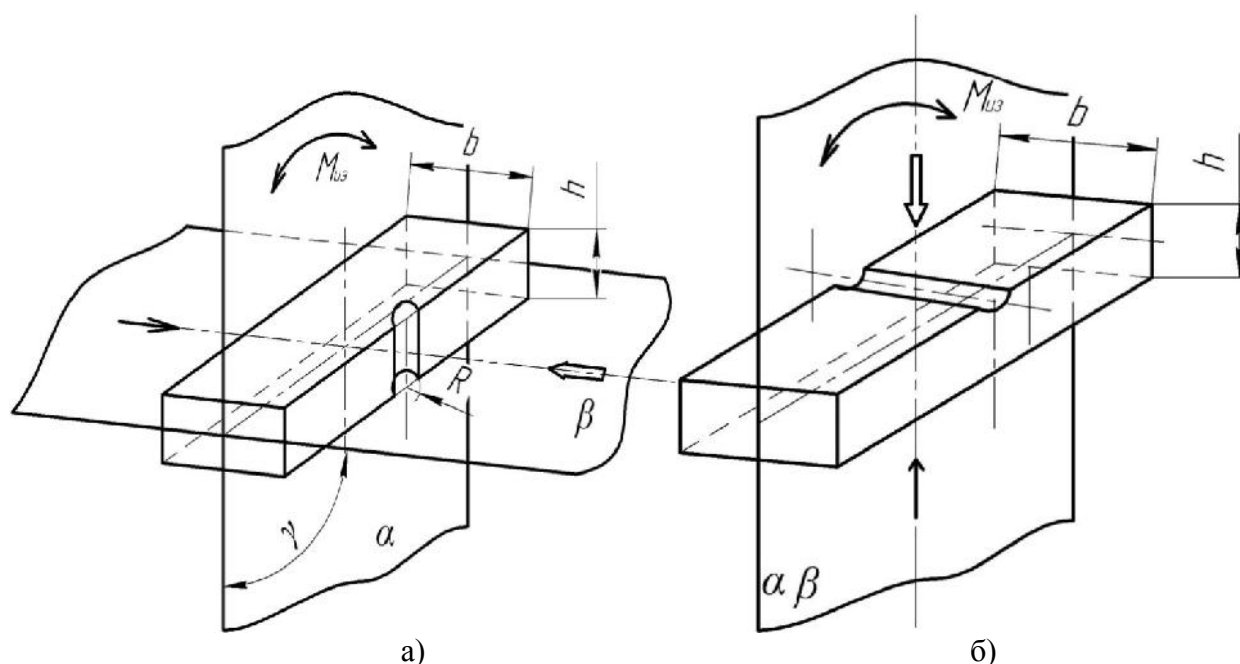
Рис. 1. Схемы предварительной деформации изгибающим моментом ( M_{из} ) и при испытании на ударный изгиб: → направление удара маятничкового копра, → направление распространения трещины в образце, а – вариант А, б – вариант Б.
