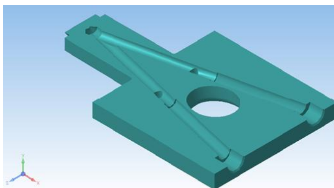
Рис. 6. БЗ в сечении, окончательная версия (показаны каналы для охлаждающей жидкости)
