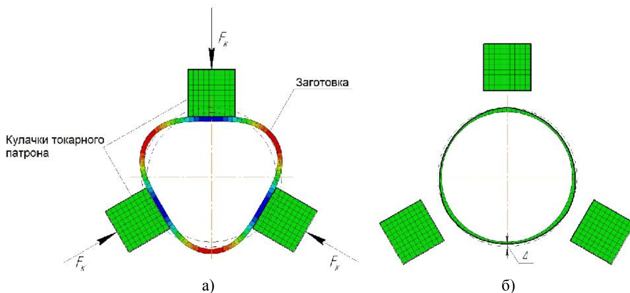
Рис. 1. Эскиз точения тонкостенной детали
