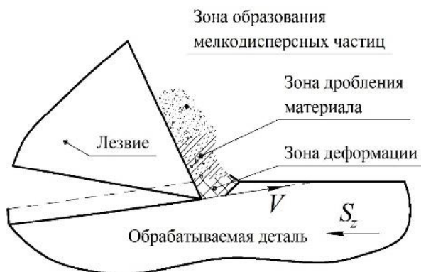
Рис. 1. Предполагаемая модель образования стружки
