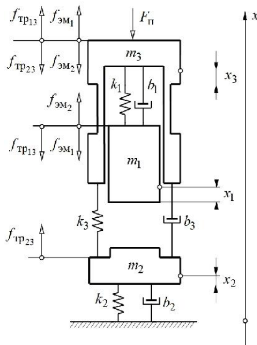
Рис. 2. Расчетная динамическая схема механической системы
