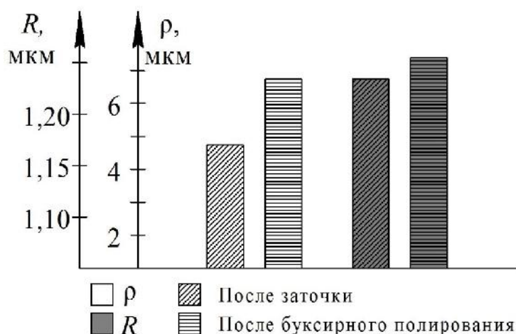
Рис. 4. Изменение радиуса округления и шероховатости режущих кромок концевых фрез после буксирного полирования в абразиве M 5/300
