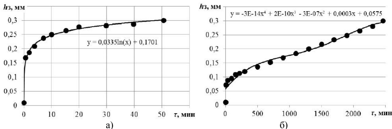
Рис. 2. Кривые износа режущего инструмента в зависимости от времени обработки: а) при V = 51,5 м/с; S_z = 0,1 мм/зуб; t = 0,5 мм; б) при V = 19,2 м/с; S_z = 0,1 мм/зуб; t = 0,5 мм
