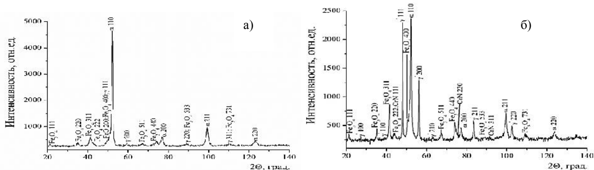
Рис. 1. Фрагменты рентгеновских дифрактограмм ( \text{CoK}\alpha ) от поверхностных слоев покрытия из стали 40X13, после различных режимов обработки: а – исходное состояние; б – ионно-лучевое азотирование при 870 К
