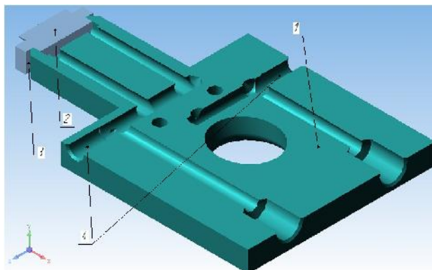
Рис. 4. Разъёмная конструкция БЗ с каналами для охлаждающей жидкости: 1 – знак большой; 2 – заглушка знака большой; 3 – место под сварку; 4 – технологические отверстия
