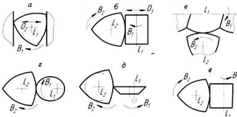
Рис. 3. Схемы профилирования методом обката при разделенных ( a, б ) и совмещенных ( в – e ) движениях профилирования и резания
