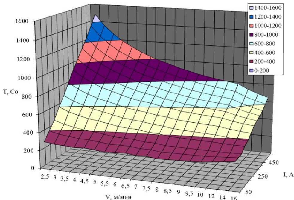
Рис. 3. Зависимость расчетных значений температуры в микрообъеме обрабатываемого поверхностного слоя от режимов ФЭМ
