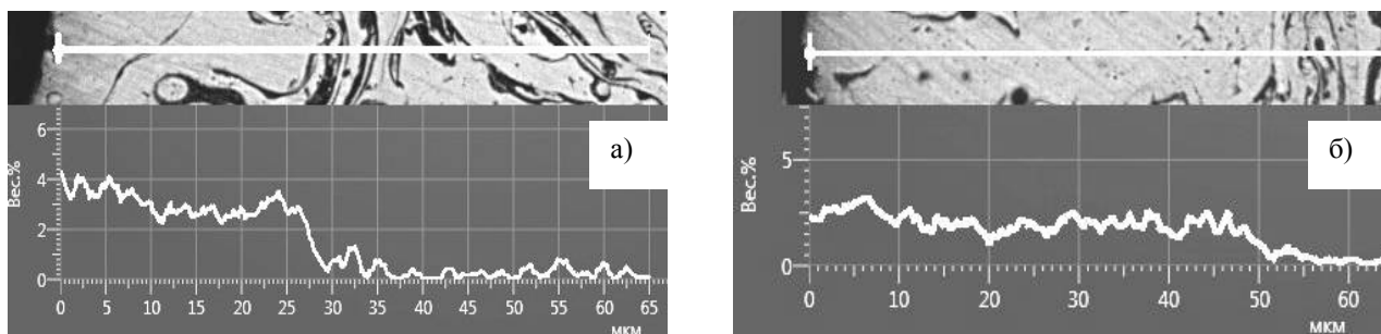
Рис.3. Распределение азота по глубине газотермического покрытия из стали 40X13, прошедшего ионно-лучевое азотирование при 870 К (3 часа):
