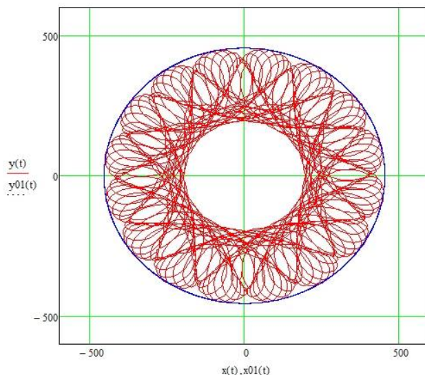
Рис. 1. Пример траектории движения заготовки, воспроизводимой при буксирном полировании
