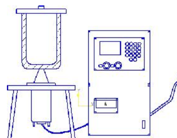
Рис. 3. Схема установки
