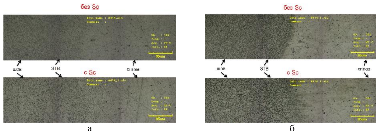
Рис. 2. Фотография поперечного шлифа сварного шва и основного сплава без Sc и с Sc: а) система Al-Mg-Li, сплав 1420; б) система Al-Cu-Li, сплав 1441.
