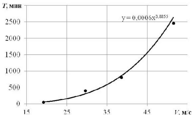
Рис. 3. Зависимость периода стойкости режущего инструмента от скорости резания
