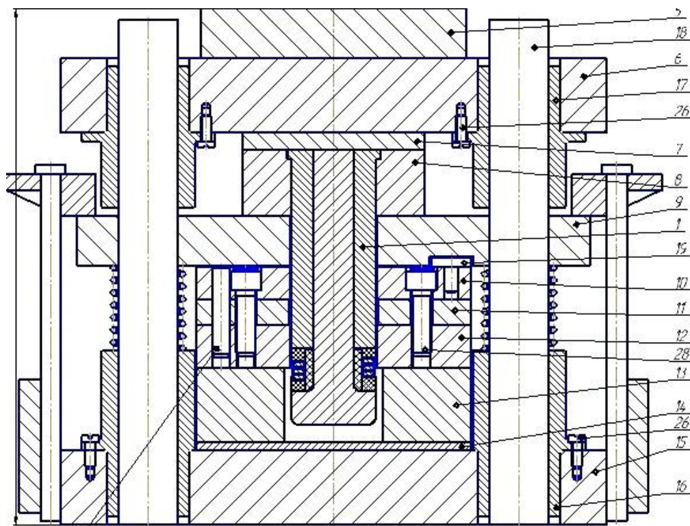
Рис. 3. Сборочный чертеж штампа для операции «вытяжка – обрезка припуска»:
