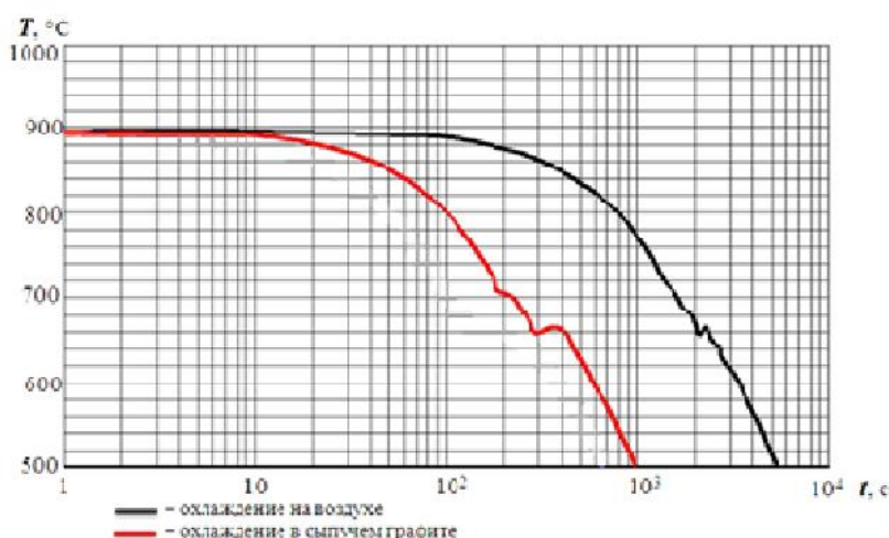
Рис.1. Изменение температуры наплавленных образцов при различных условиях охлаждения после термообработки
