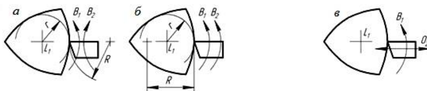
Рис. 1. Рациональные схемы профилирования НП методом следа при полигональном (а, б) и некруглом точении (в)
