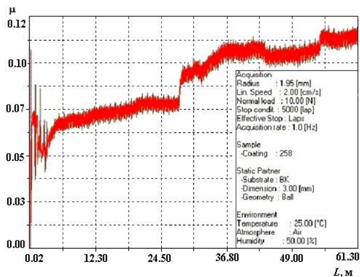
Рис. 2. Зависимость коэффициента трения \mu от длины трека L трибологических испытаний. На вставке приведены условия трибологических испытаний
