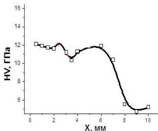
Рис. 1. Профиль микротвердости системы «наплавленный слой / сталь»
