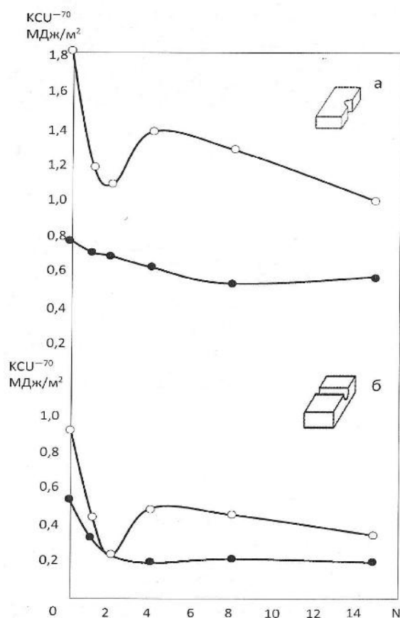
Рис. 2. Изменение ударной вязкости в зависимости от числа циклов изгиба (N):
