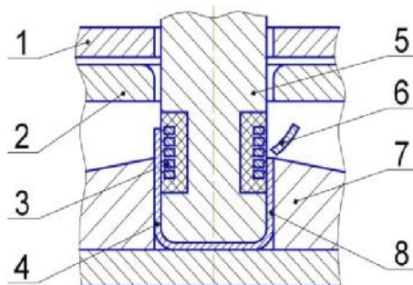
Рис. 2. Схема процесса вытяжки и обрезки припуска:
