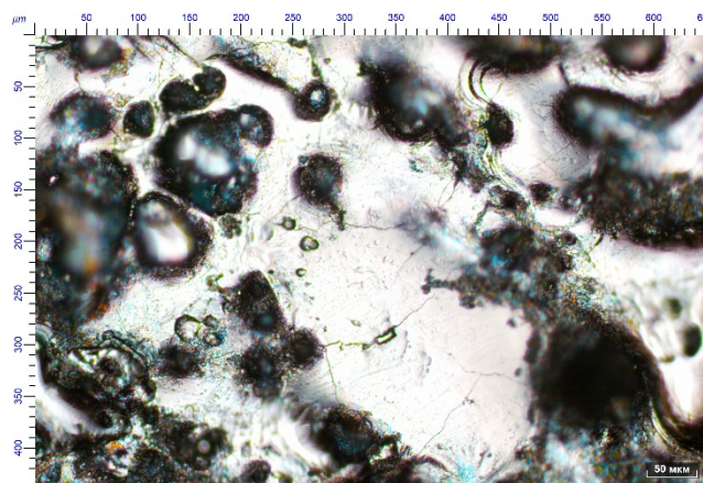
Рис. 8. Поверхность электрода после КПЭЭО на максимальном режиме при увеличении \times 500 (а) и \times 300 (б)
