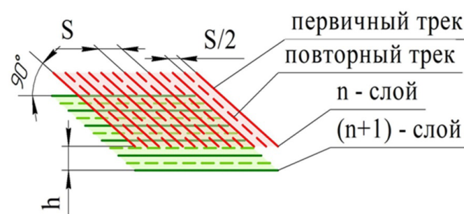
Рис. 5. Стратегия сканирования IV ( \angle 90^\circ п.п.)
