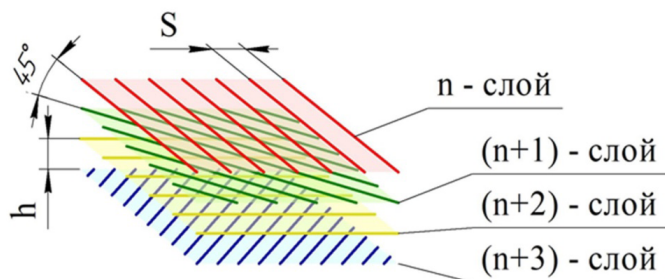
Рис. 3. Стратегия сканирования II ( \angle 45^\circ )
