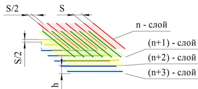
Рис. 4. Стратегия сканирования III ( \angle 90^\circ S/2 )
