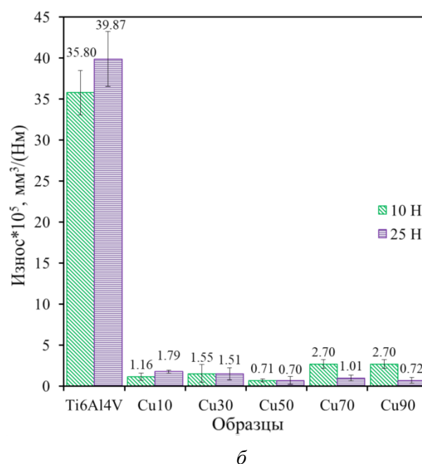
Рис. 5. Коэффициент трения (а) и износ (б) Cu-Ti-покрытий и сплава Ti6Al4V в растворе SBF при различных нагрузках
